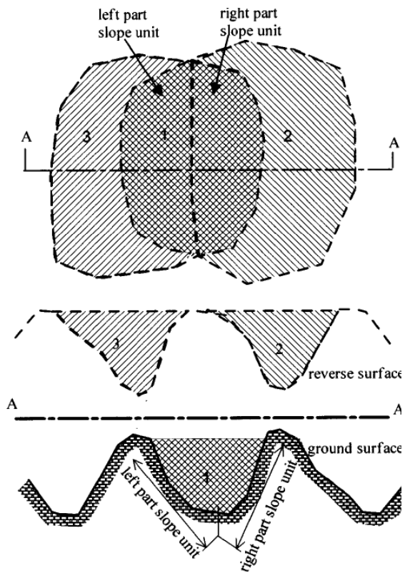
圖 4. 由集水區 DEM 與反轉集水區 DEM 劃分邊坡單元 (Xie, et al. 2003)
