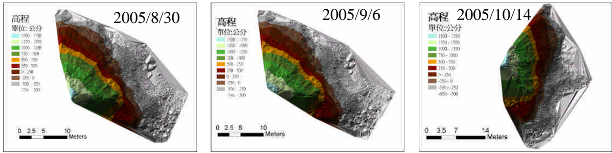
圖 9. 三次數值掃描所建立之不規則網格數值高程模型
