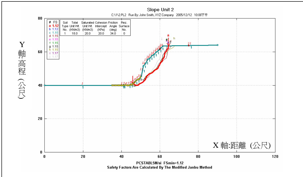
圖 12. Slope unit 2 之穩定性分析結果
