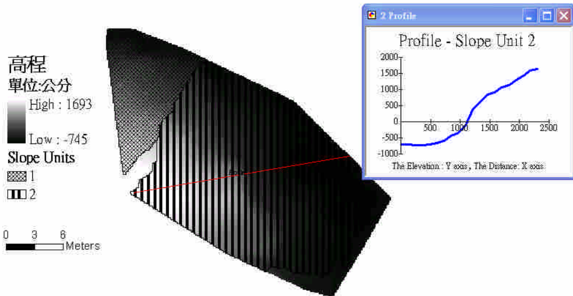
圖 6. 經由繪製剖面線產生地形剖面圖
