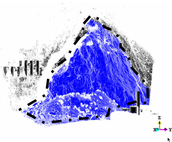
圖 2. 資料處理前與資料處理後之三維立體圖
