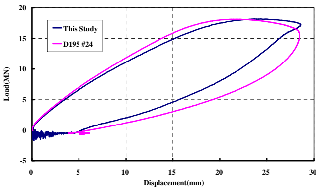
圖 8 D195 #24 :「This Study」與「D195 #24」載重-變位關係圖
