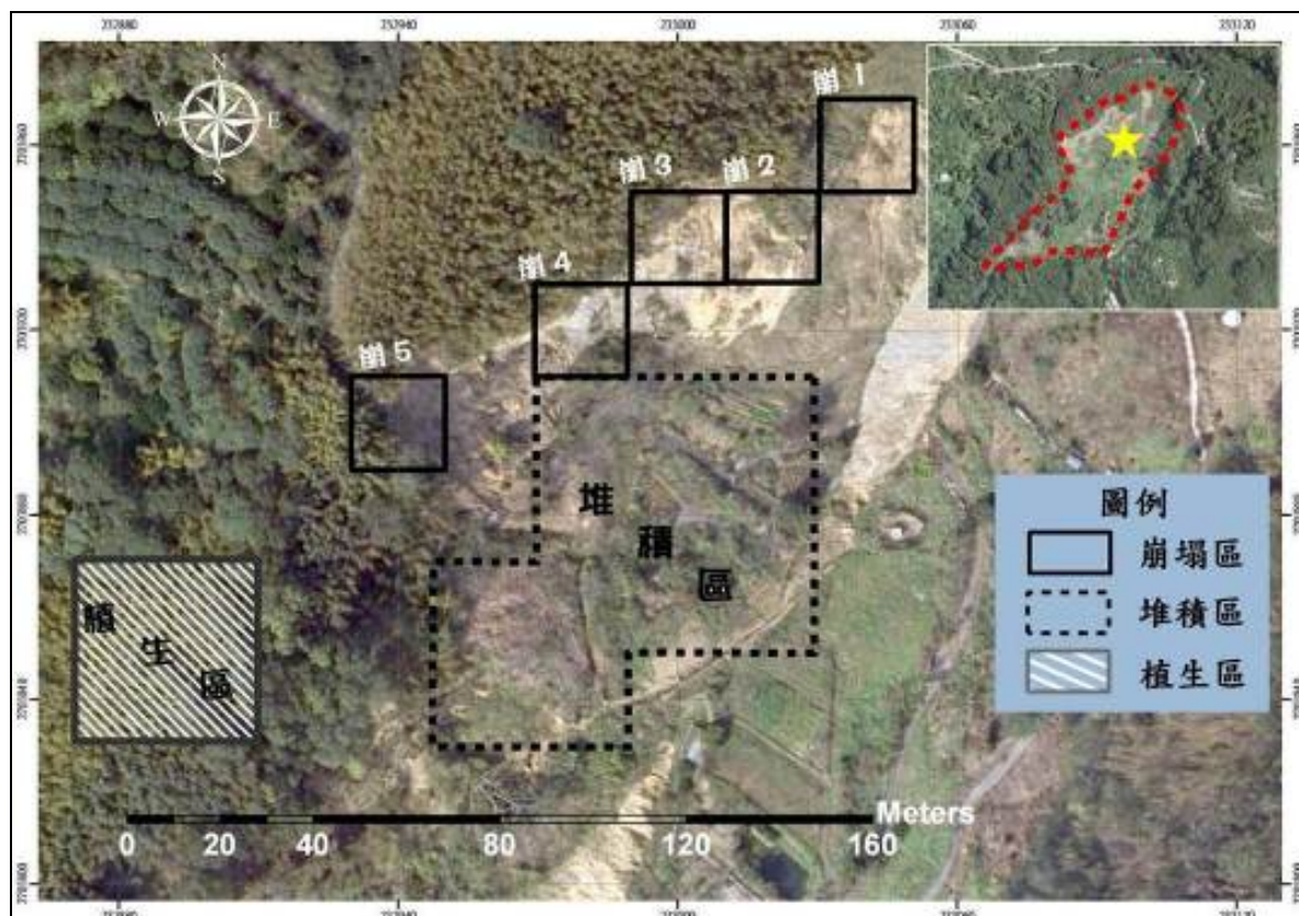
圖 11 邊坡植生變遷監測分析區位
